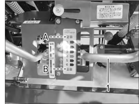
(1) 식부깊이 조절 레버 (A) 얇음 (B) 깊음
