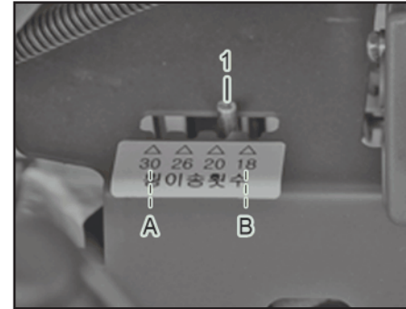
(1) 횡 이송 변환 레버 (A) 횡 이송 30회 (B) 횡 이송 18회
