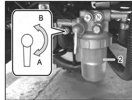
(1) 연료 필터 (A) 개 (B) 폐 (2) 유수 분리기 (A) 개 (B) 폐
