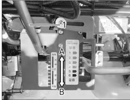
(1) 식부분수 조절 레버 (A) 많음 (B) 적음
